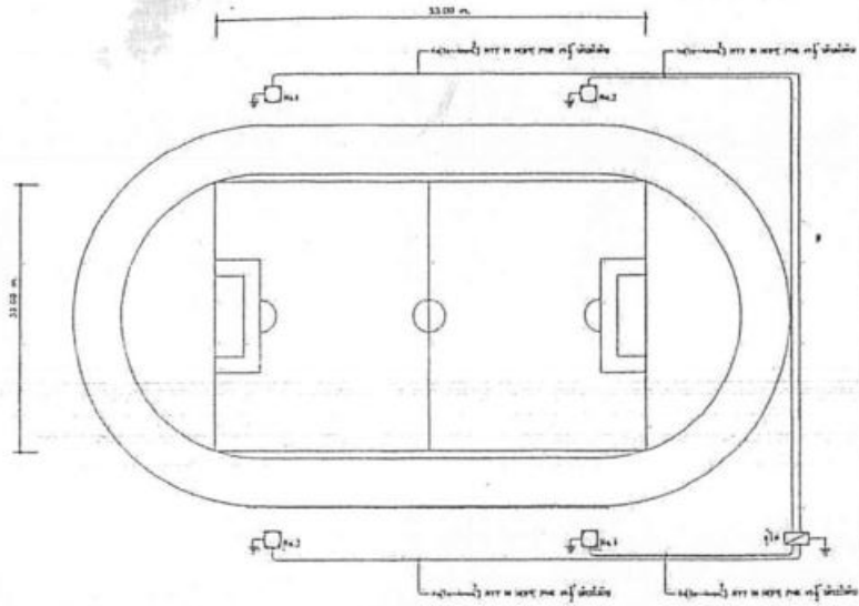
แบบแสดงตำแหน่งโคมไฟเสาสูงสนาม SCALE 1:1,500
